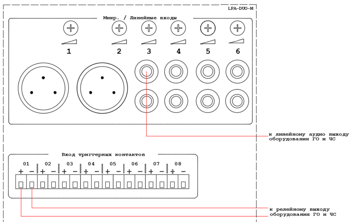
Рис. 2.3. Схема подключения сигналов ГО и ЧС к LPA-DUO
