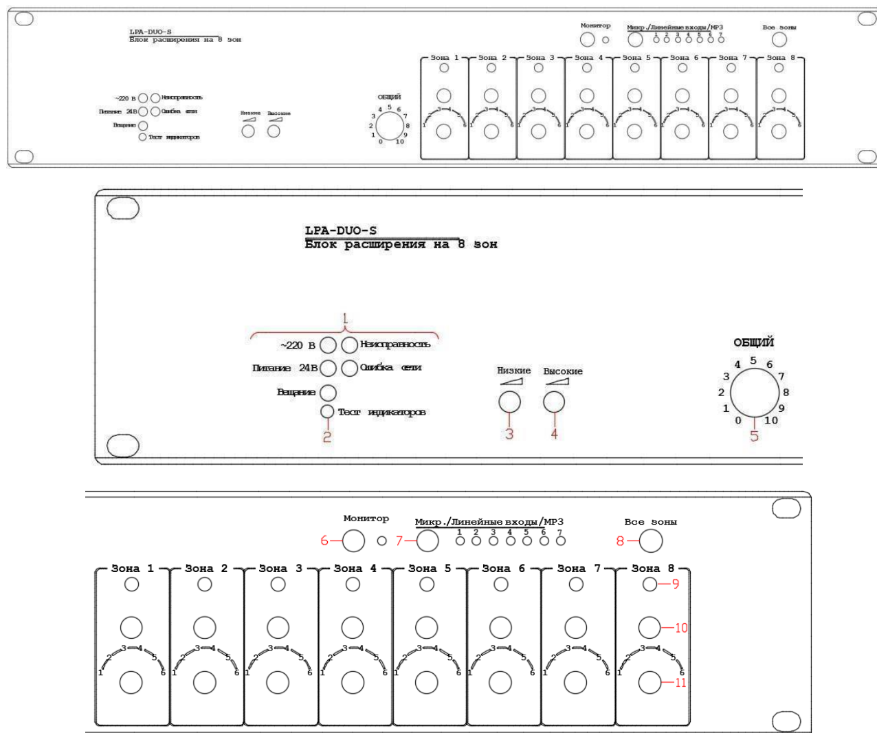
Рис. 2.3. Блок расширения LPA-DUO-S (передняя панель)
