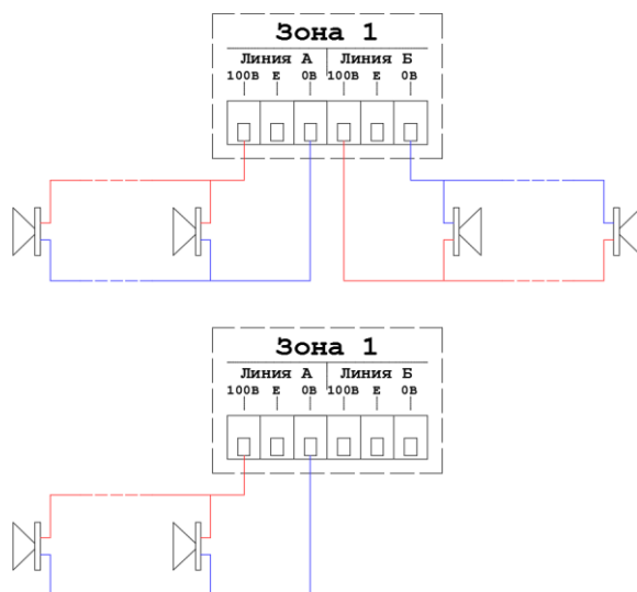
Рис. 2.3. Схема подключения трансляционных линий к LPA-DUO
