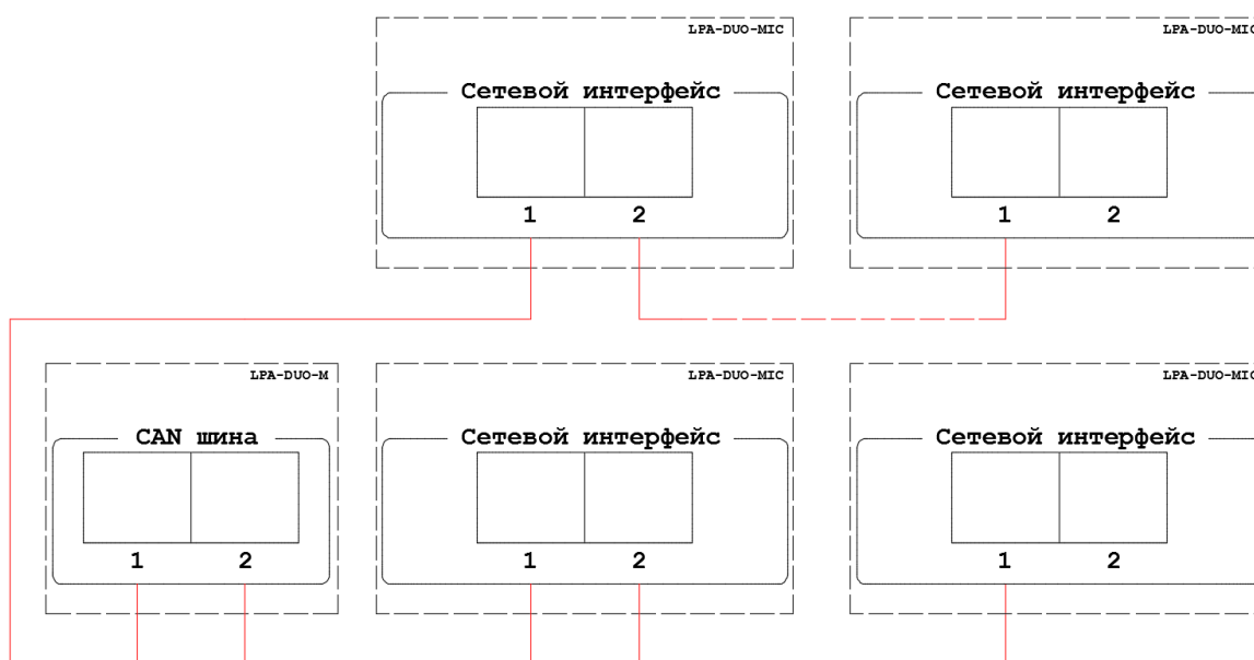
Рис. 2.3. Схема подключения удаленных микрофонных консолей к LPA-DUO
