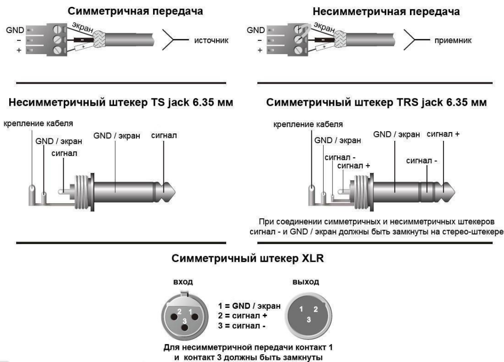
Рис. 1.1. Назначение контактов разъемов
