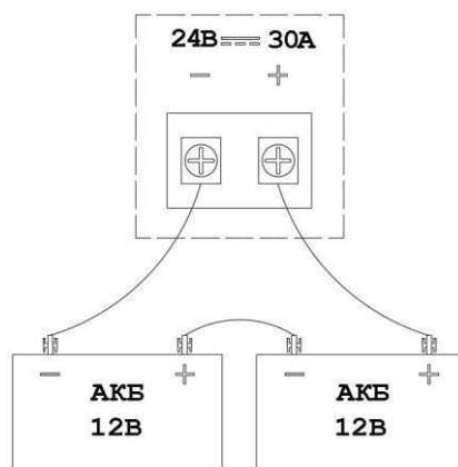
Рис. 2.3. Схема подключения АКБ к LPA-DUO
