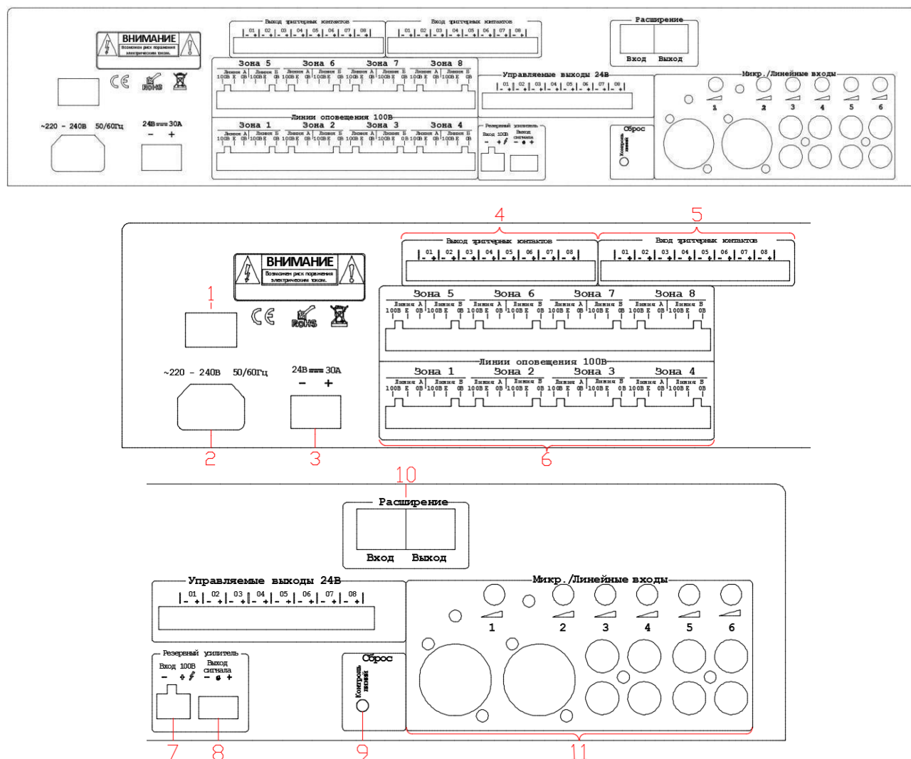
Рис. 1.2. Блок расширения LPA-DUO-S (задняя панель)
