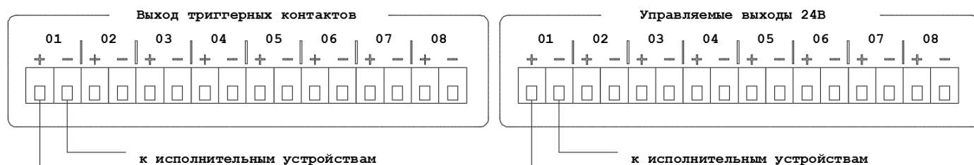
Рис. 2.3. Схема подключения внешних исполнительных устройств к LPA-DUO
