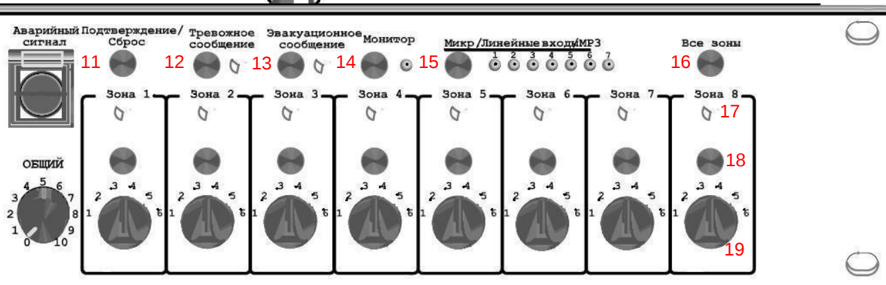
Рис. 1.1. Контроллер системы LPA-DUO-M (передняя панель)
