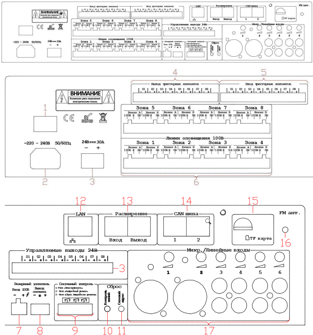
Рис. 1.1. Контроллер системы LPA-DUO-M (задняя панель)
