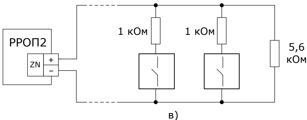
б), в) Подключение извещателей типа «Аврора-ДН, -ТН, -ДТН» с распознаванием срабатки двух извещателей в ШС. Тип ШС – «пожарный дымовой».
