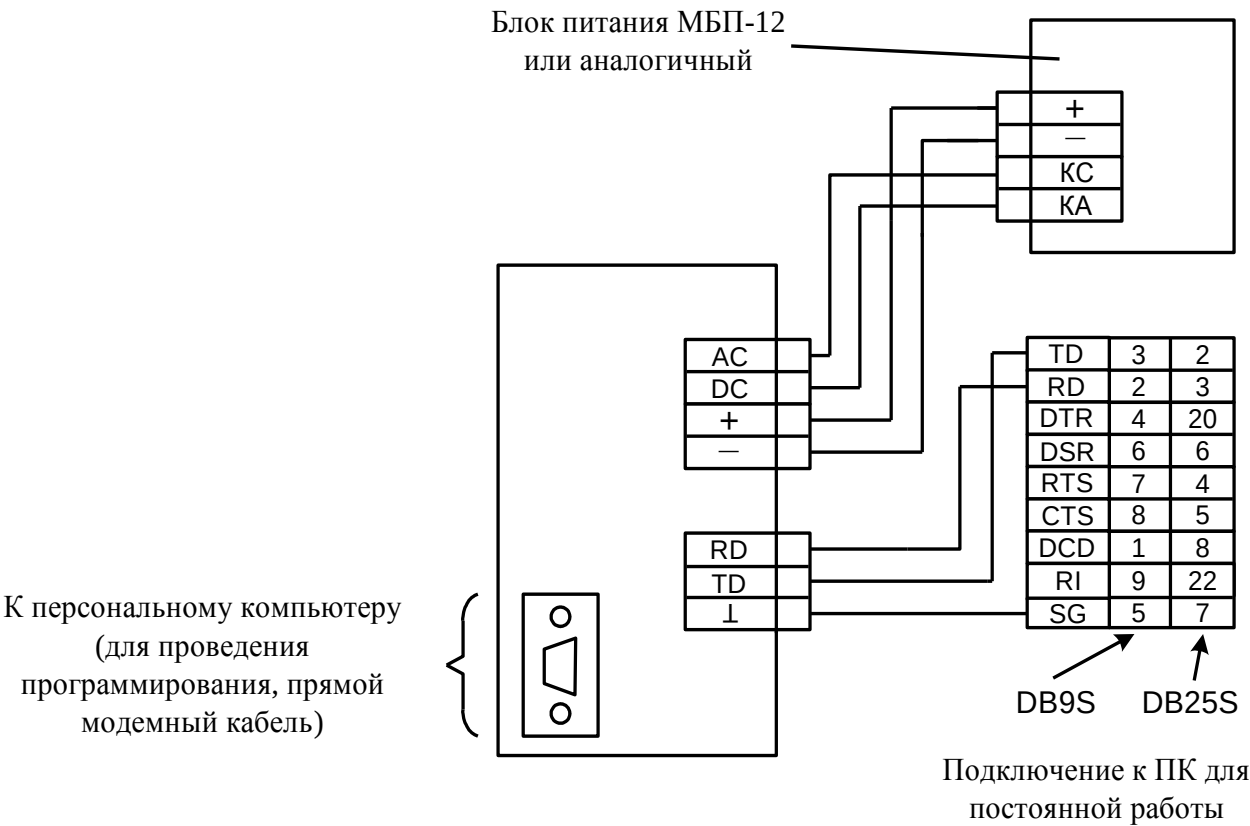
Рисунок В.6 – Схема внешних подключений РРОП-М, РРОП-М2
