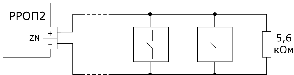
а) Подключение извещателей типа «Аврора-ДН, -ТН, -ДТН» без распознавания срабатки двух извещателей в ШС. Тип ШС – «пожарный дымовой».
