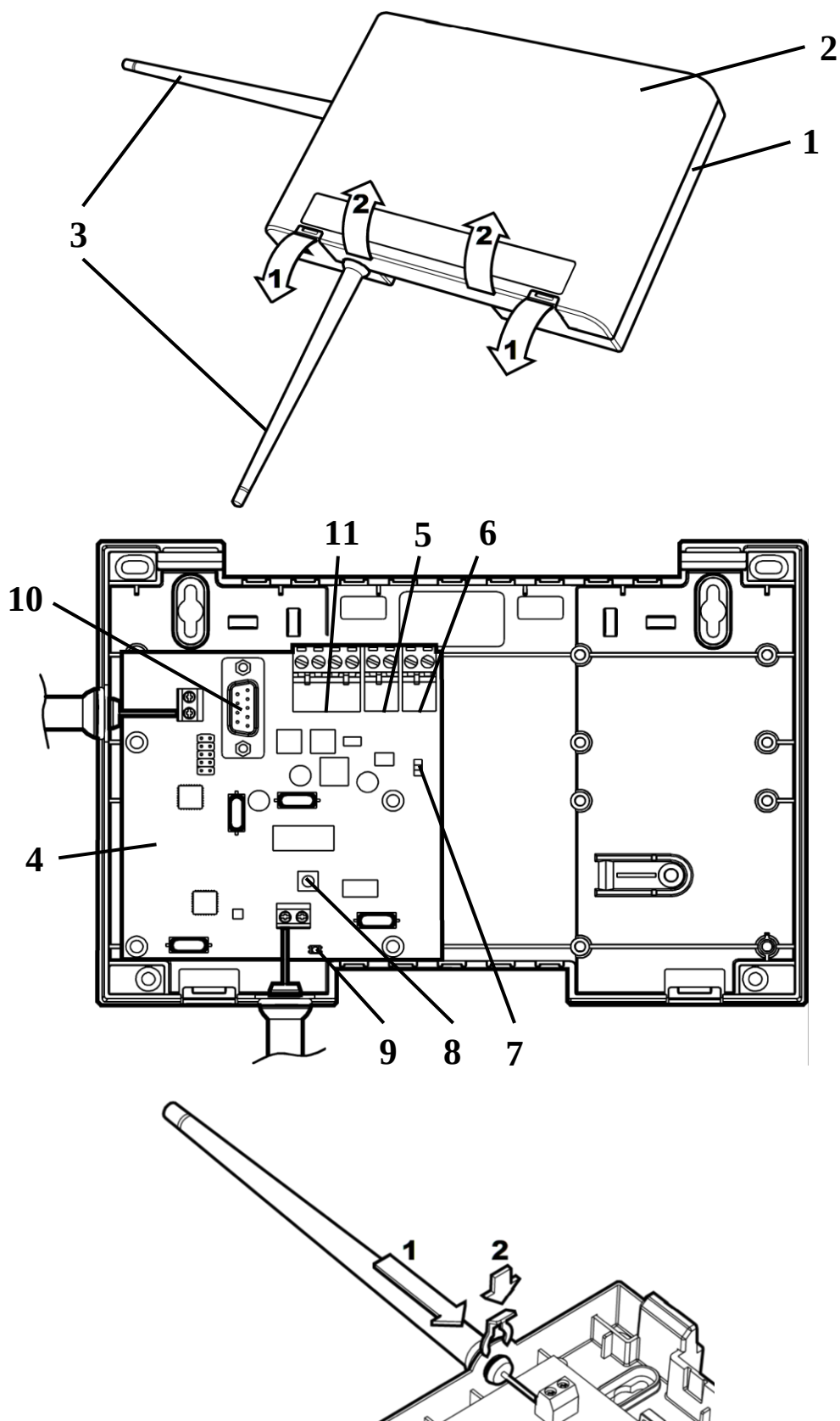
Рисунок Б.36 – Внешний вид РРОП-М2
