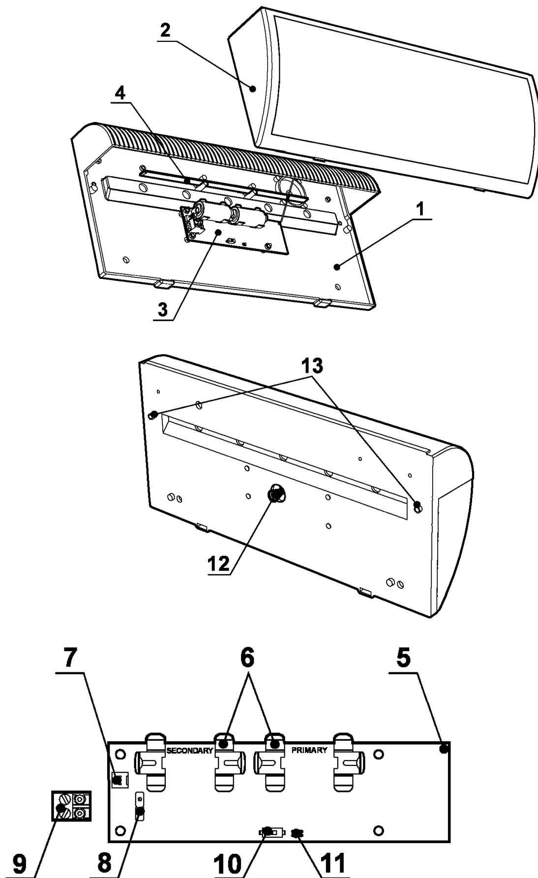
Рисунок Б.21 – Внешний вид устройства "Табло-Р"
