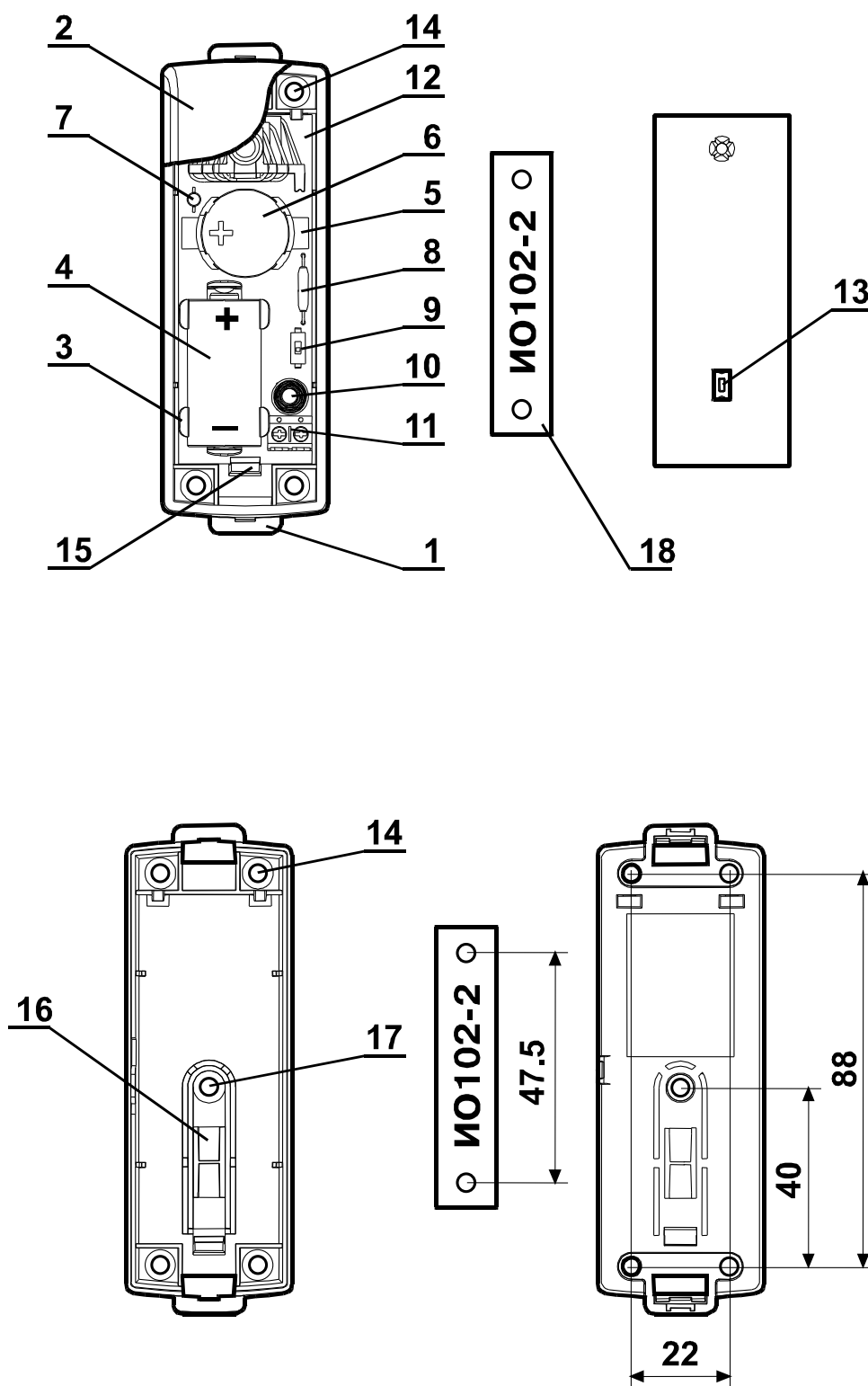
Рисунок Б.13 – Внешний вид ИО РИГ
