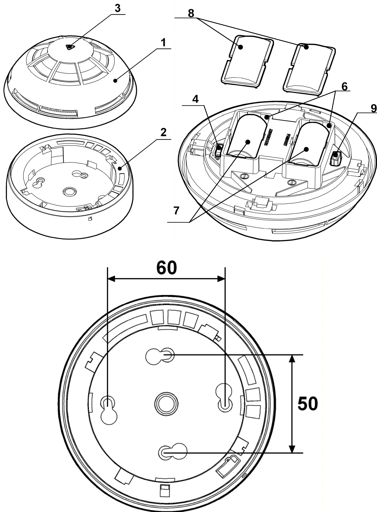
Рисунок Б.20а – Внешний вид устройства "Аврора-ДОР"
