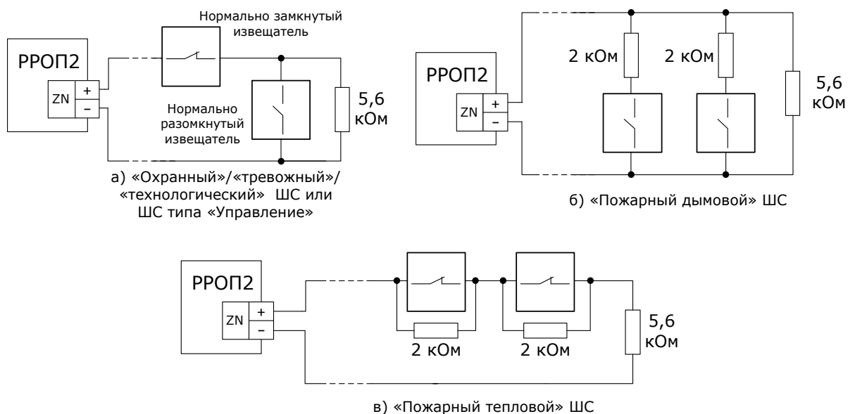
Рисунок В.4 – Подключение в ШС РЕОП2 извещателей с выходом типа "сухой контакт"
