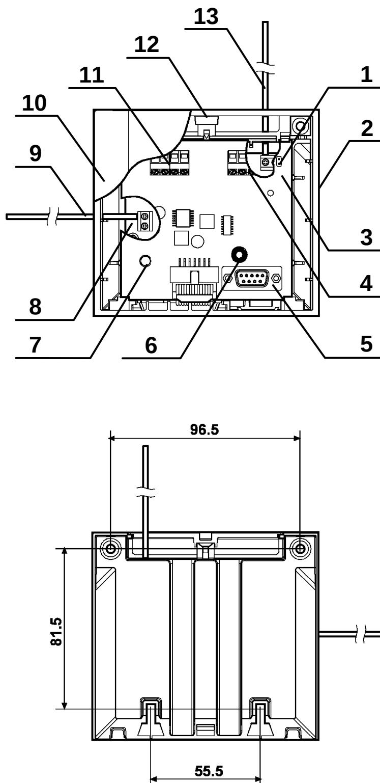
Рисунок Б.3 – Внешний вид РРОП-М
