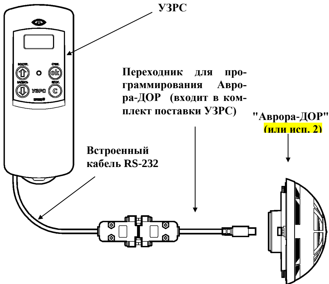
Рисунок В.23 – Подключение УЗРС для программирования речевых сообщений в устройства "Аврора-ДОР", "Аврора-ДОР исп.2"
