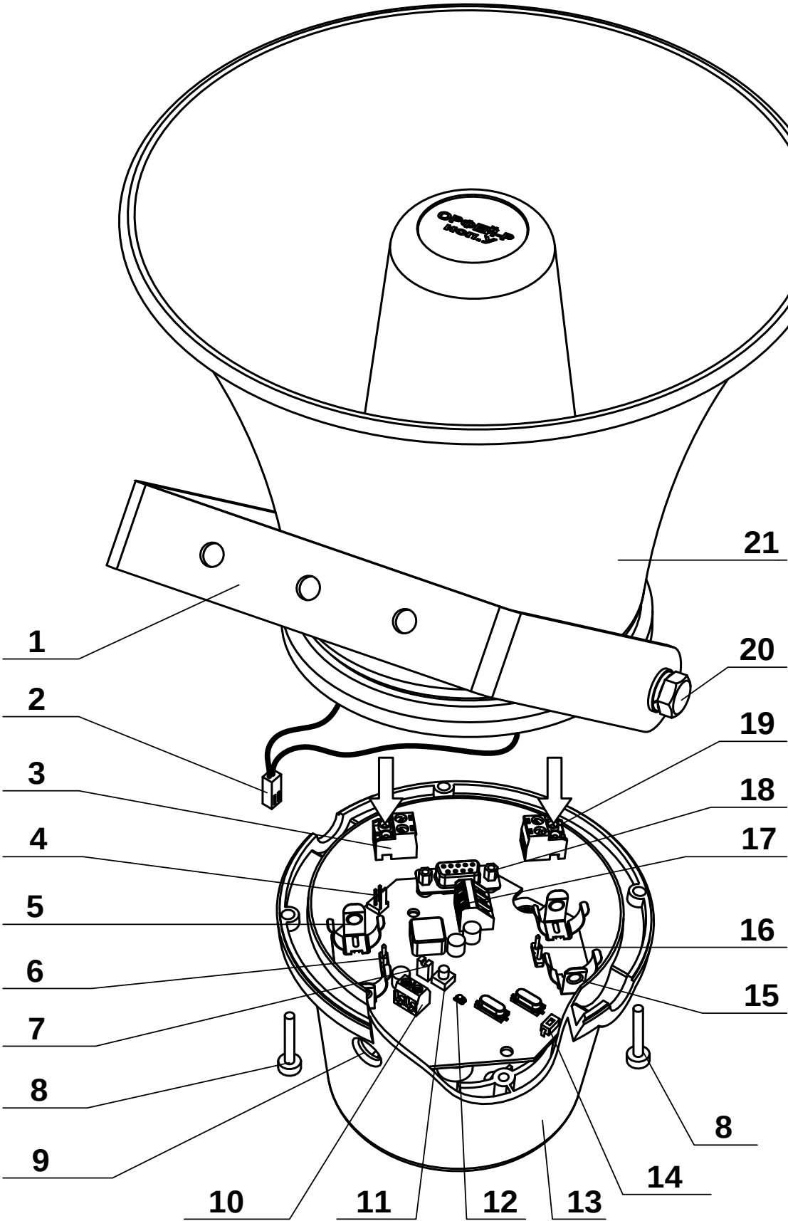
Рисунок Б.26 – Внешний вид устройства "Орфей-Р исп. У"
