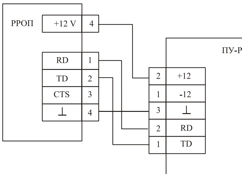
Рисунок В.11 – Схема стационарного подключения ПУ-Р (ПУП-Р) к ПРОП
