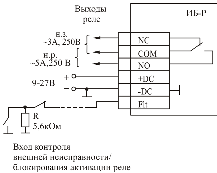
Рисунок В.8 – Схема подключения ИБ-Р
