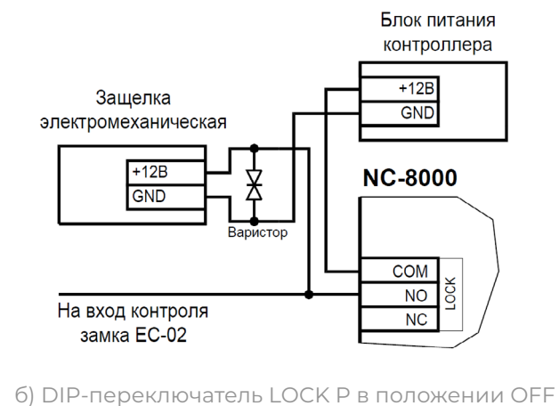
Рисунок 5. Контроль состояния замка, запираемого напряжением
