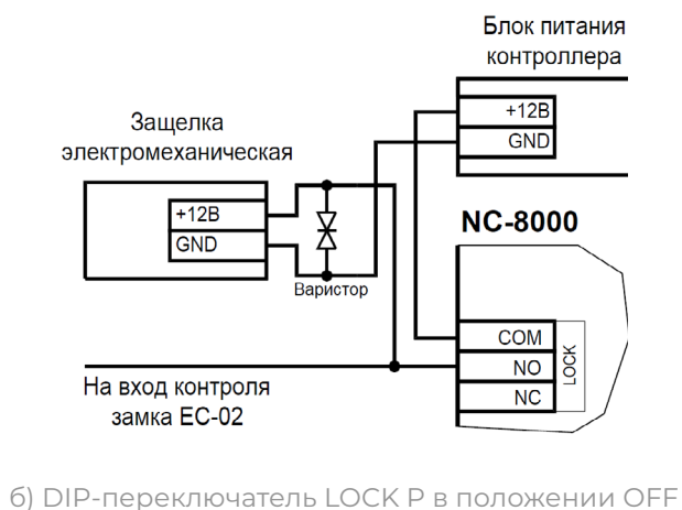
Рисунок 4. Контроль состояния замка, запираемого напряжением
