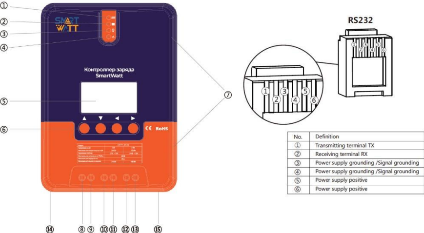
Рисунок 1-1. Внешний вид контроллера и разъемы
