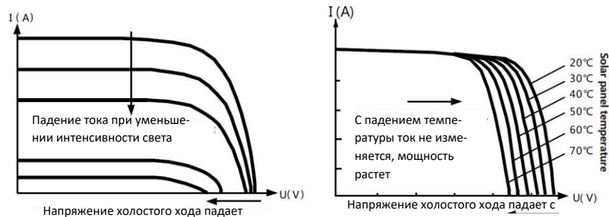
Рисунок 1-3. Зависимость выходных параметров модуля от освещенности
