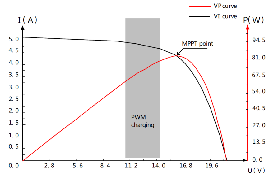
Рисунок 1-2. График выходных параметров солнечного модуля
