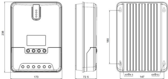
MPPT2430/MPPT2440 Габариты: 238×173×72,5мм Монтажные отверстия: 180×147мм Диаметр отверстий: ф3мм Кабель: макс. 8мм 2
