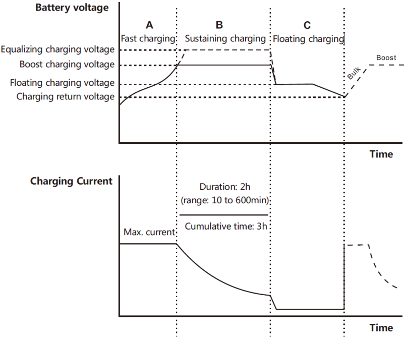
Рисунок 1-5. График этапов заряда аккумулятора
