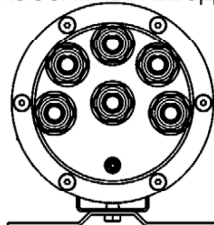
Рисунок 3 – Стандартное расположение кабельных вводов
