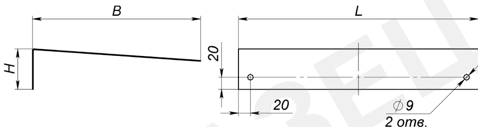
Рис.1 Установочные и габаритные размеры
