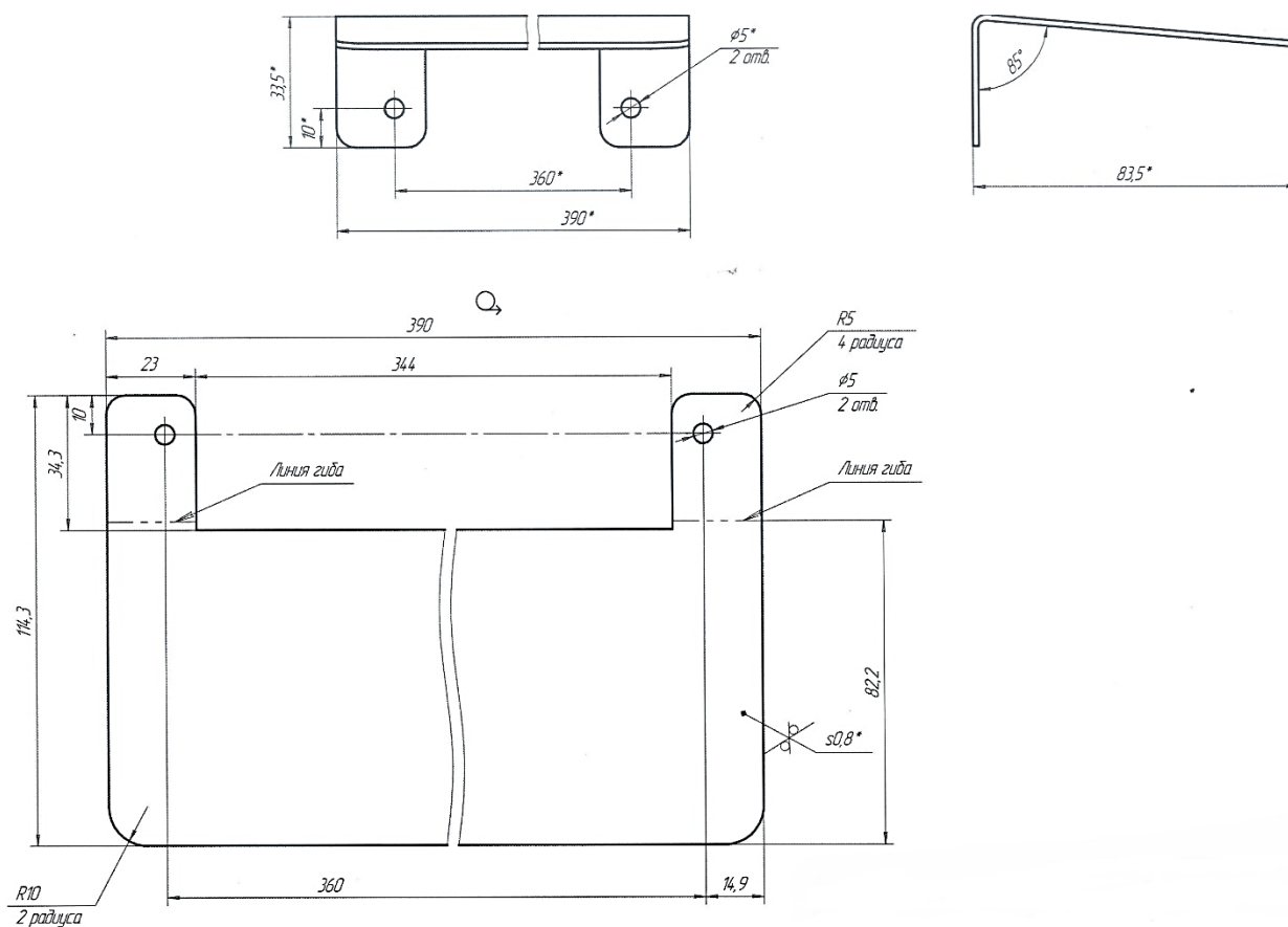
Рисунок 4 - Габаритный чертеж СЗК-32
