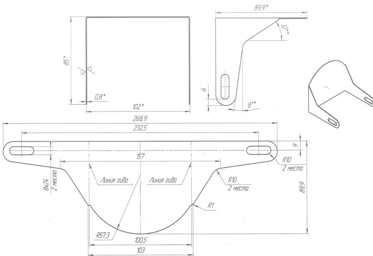
Рисунок 3 - Габаритный чертеж – СЗК-25
