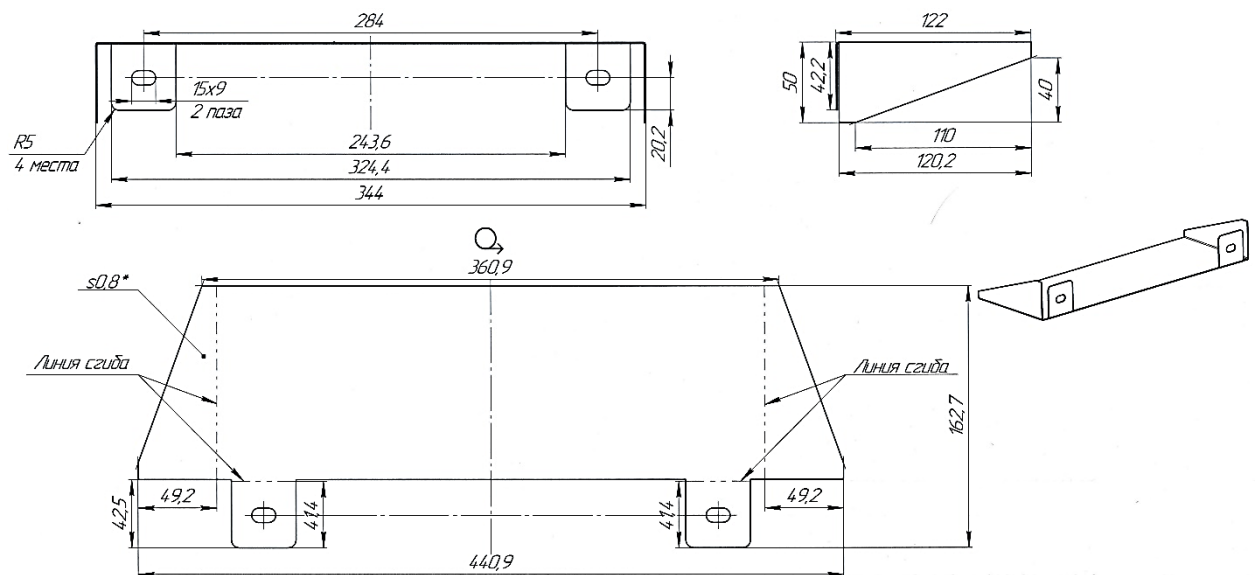
Рисунок 5 - Габаритный чертеж – СЗК-34
