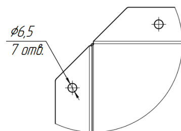
Рис.3 Диаметр крепежных отверстий.
