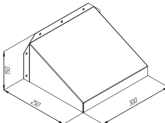
Рис.2 Габаритные размеры 300x250x150 АЯКС
