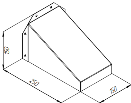
Рис.1 Габаритные размеры 150x250x150 АЯКС
