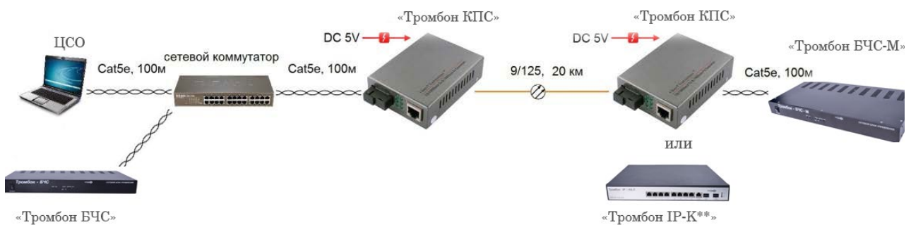
Рисунок 2 - Схема подключения для «Тромбон СДУ»
