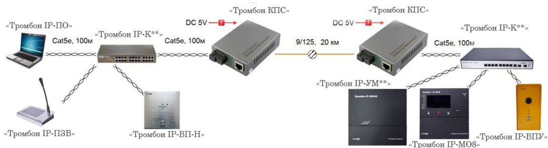
Рисунок 2 - Схема подключения для «Тромбон СДУ»
