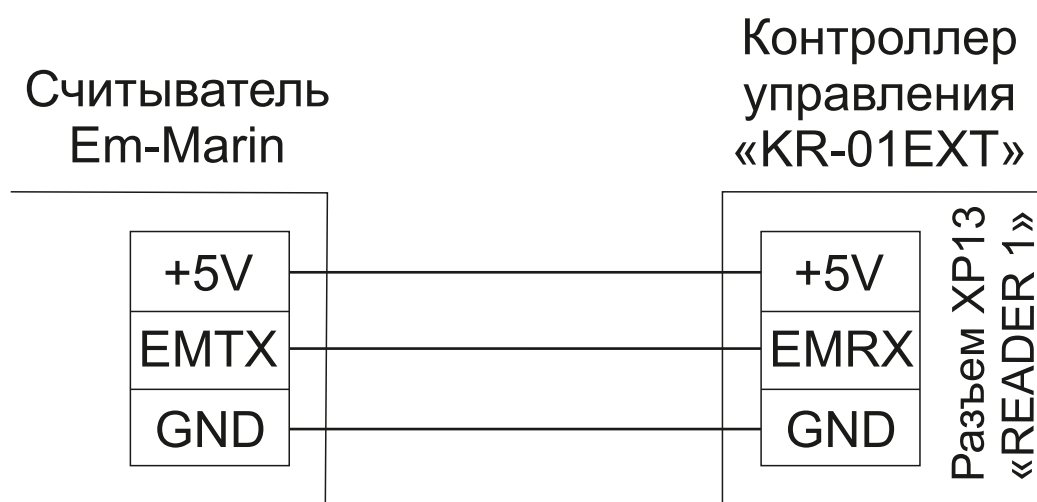
Рисунок 6.3.4 Схема подключения считывателя Em-Marin
