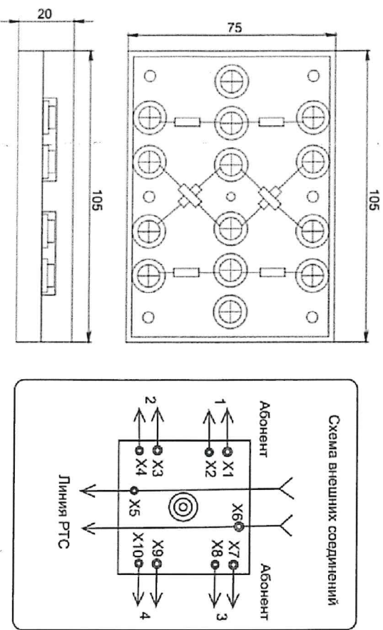
Рис.1 КОРОБКА КРА-4
