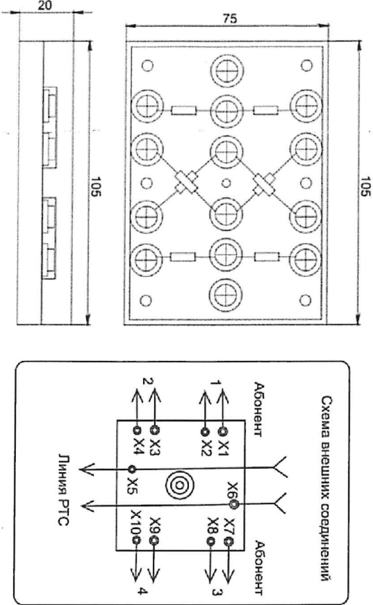
Рис.1 КОРОБКА КРА-4
