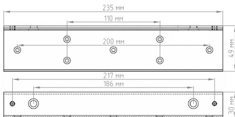
ЛКД-33-280L-68
