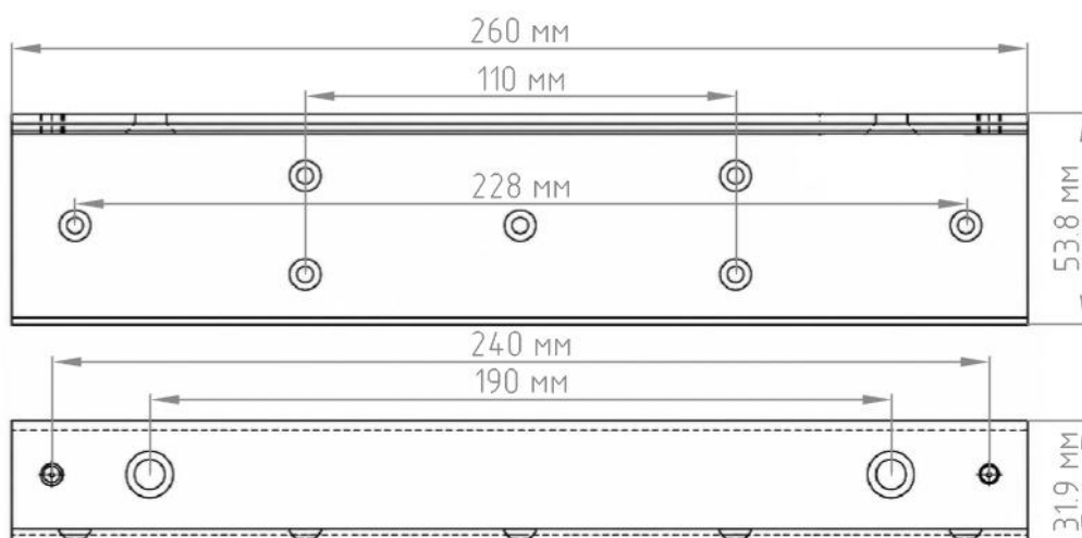
ЛКД-33-350L-68
