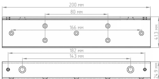
ЛКД-33-180L-68
