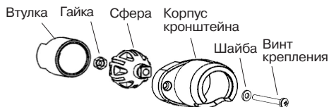
Рисунок 1 — Детали кронштейна
