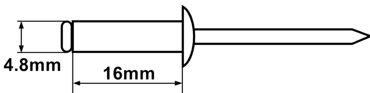
Рисунок 1-чертеж заклепки
