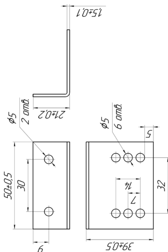
Рис.1. Габаритные и присоединительные размеры кронштейна К-20/50 АЯКС
