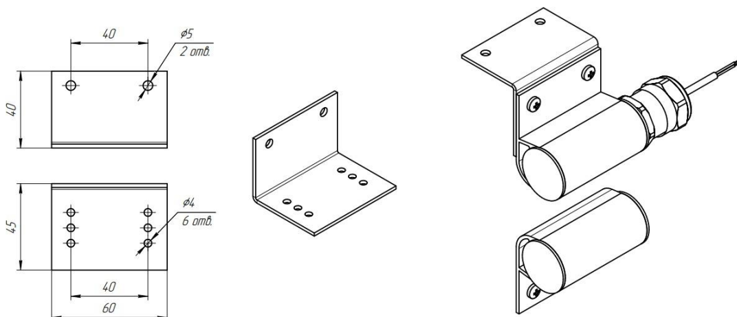
Рис.1. Габаритные и присоединительные размеры кронштейна К-100 АЯКС
