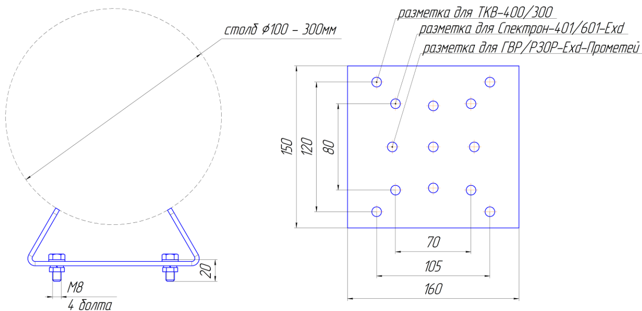
Рис. 1 – Габаритные размеры
