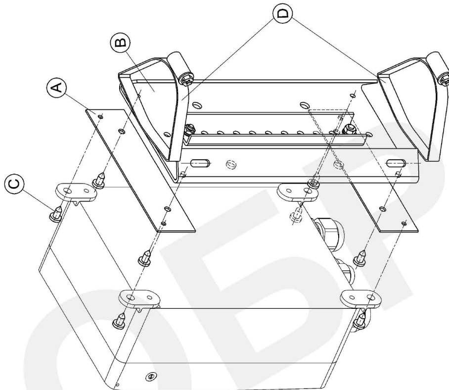
Рис.2 Монтаж кронштейна КС-1-01 для крепления КМ-1, -2, -3, БПУ-2 на квадратные и круглые опоры
