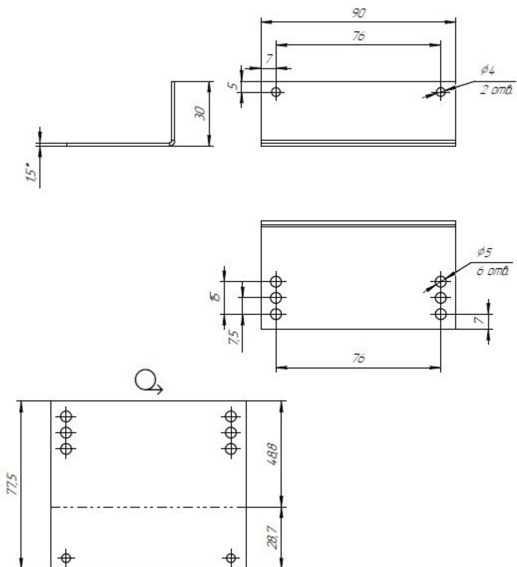
Рис.1. Габаритные и присоединительные размеры кронштейна К-ДПМ-2 АЯКС
