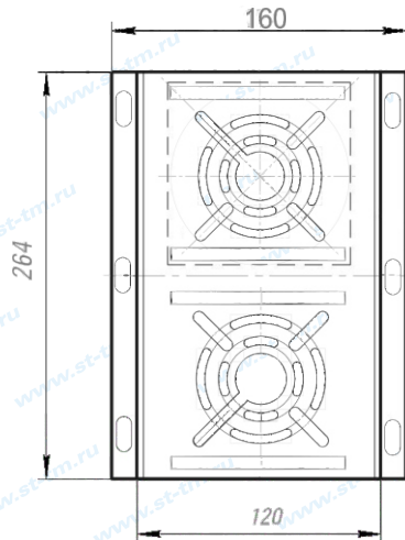
Рис.1 Габаритные размеры
