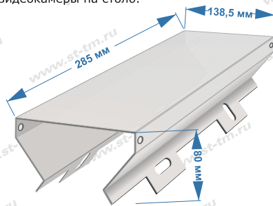
Рис.1 Габаритные размеры
