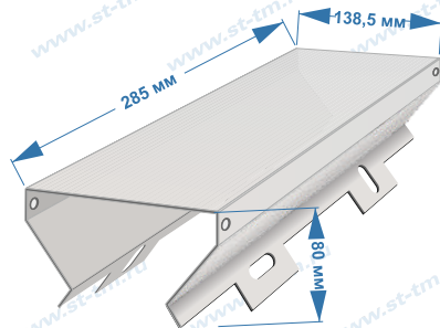
Рис.1 Габаритные размеры
