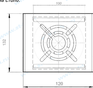
Рис.1 Габаритные размеры
