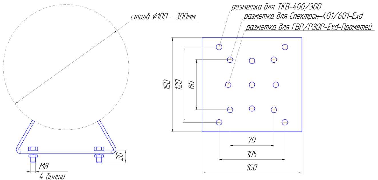
Рис. 1 – Габаритные размеры
