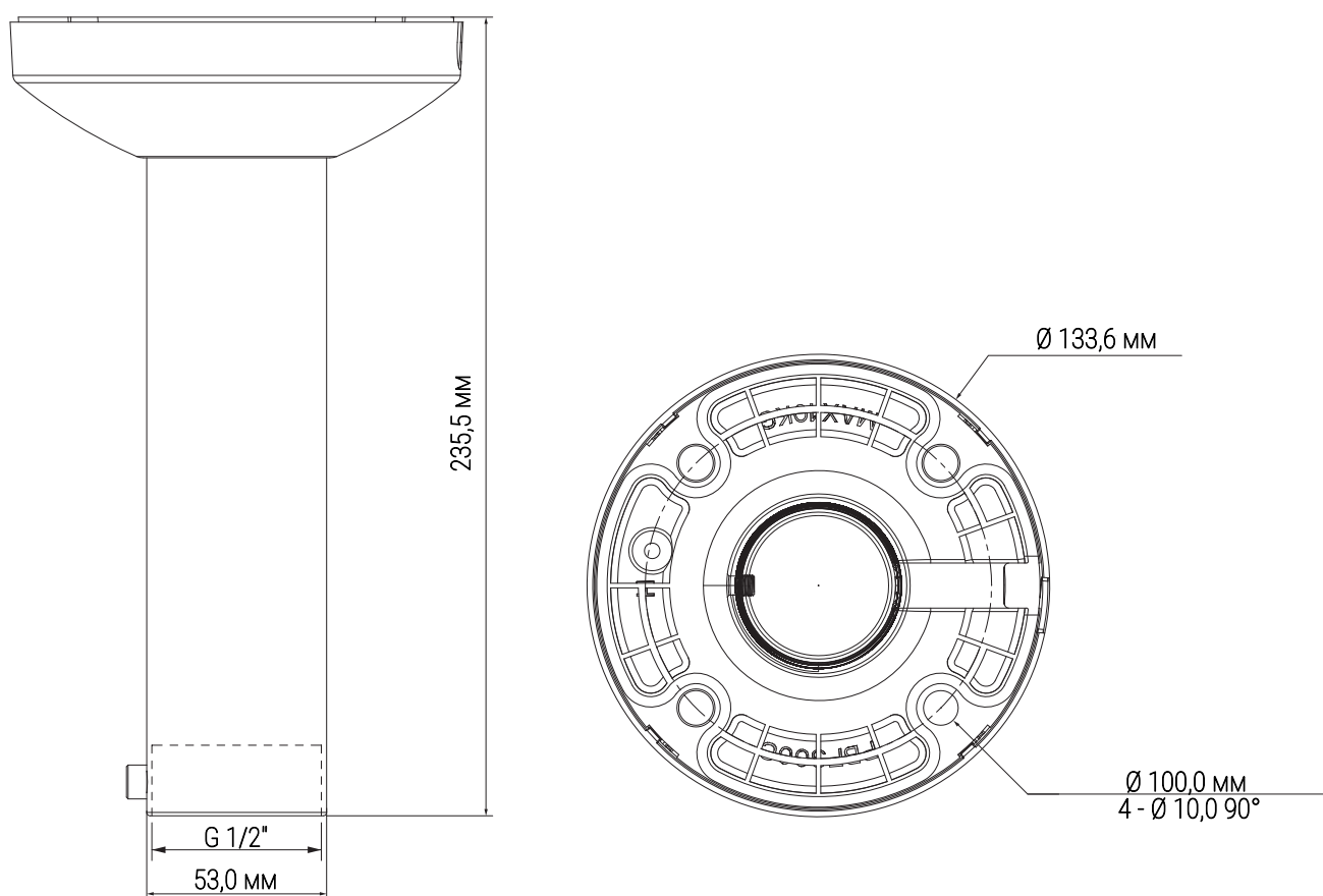
Рисунок 5.1 – Габаритные размеры
