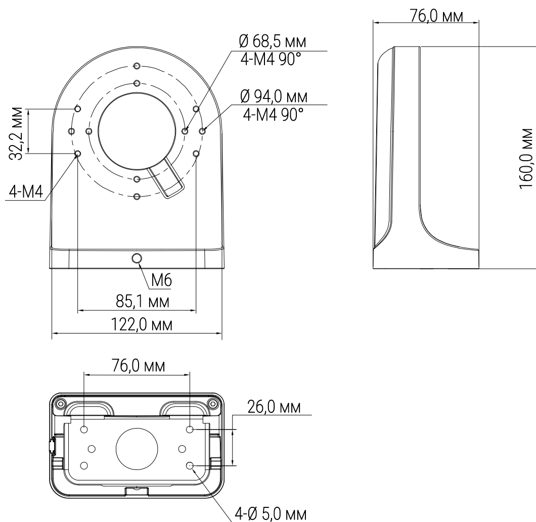
Рисунок 4.1 – Габаритные размеры
