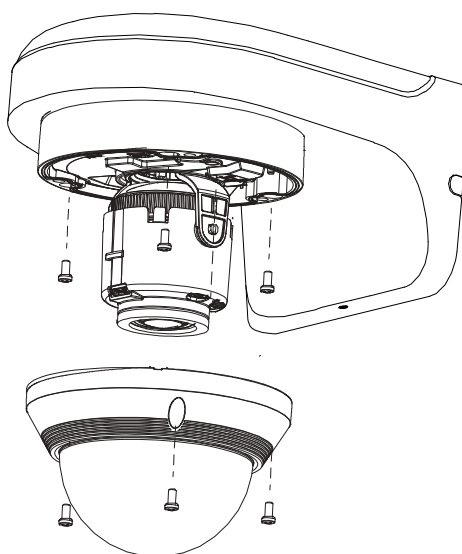
Рисунок 4.4 – Монтаж
