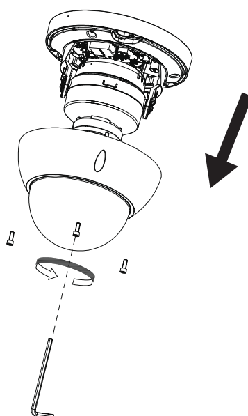
Рисунок 4.3 – Монтаж
