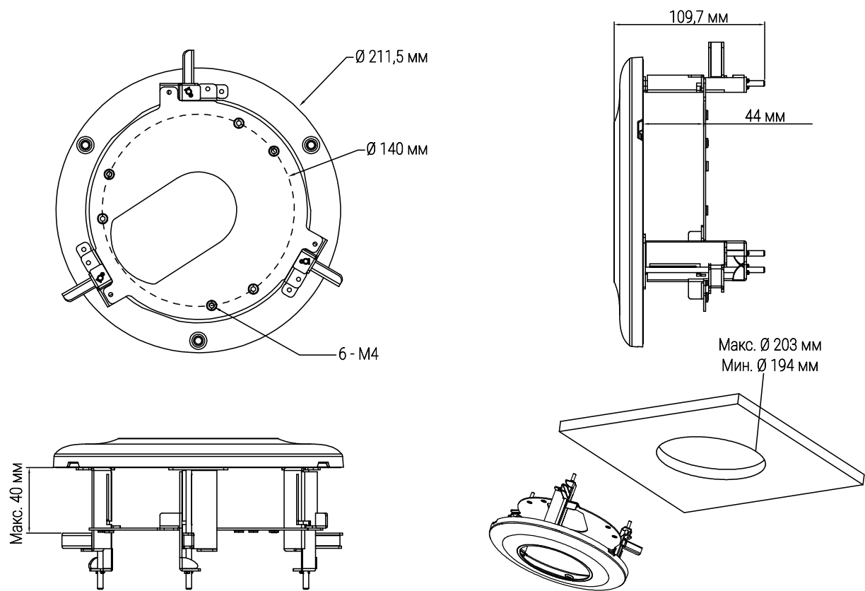
Рисунок 4.1 – Габаритные размеры
