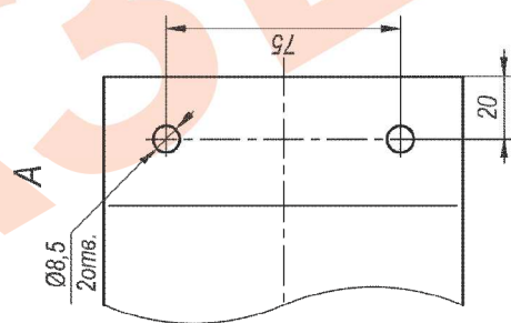
Рис.1 Установка кронштейна углового КУ-1
