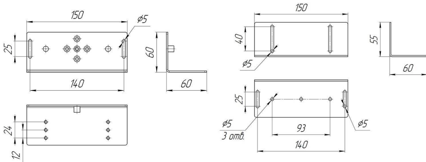
Рис.1. Габаритные и присоединительные размеры
