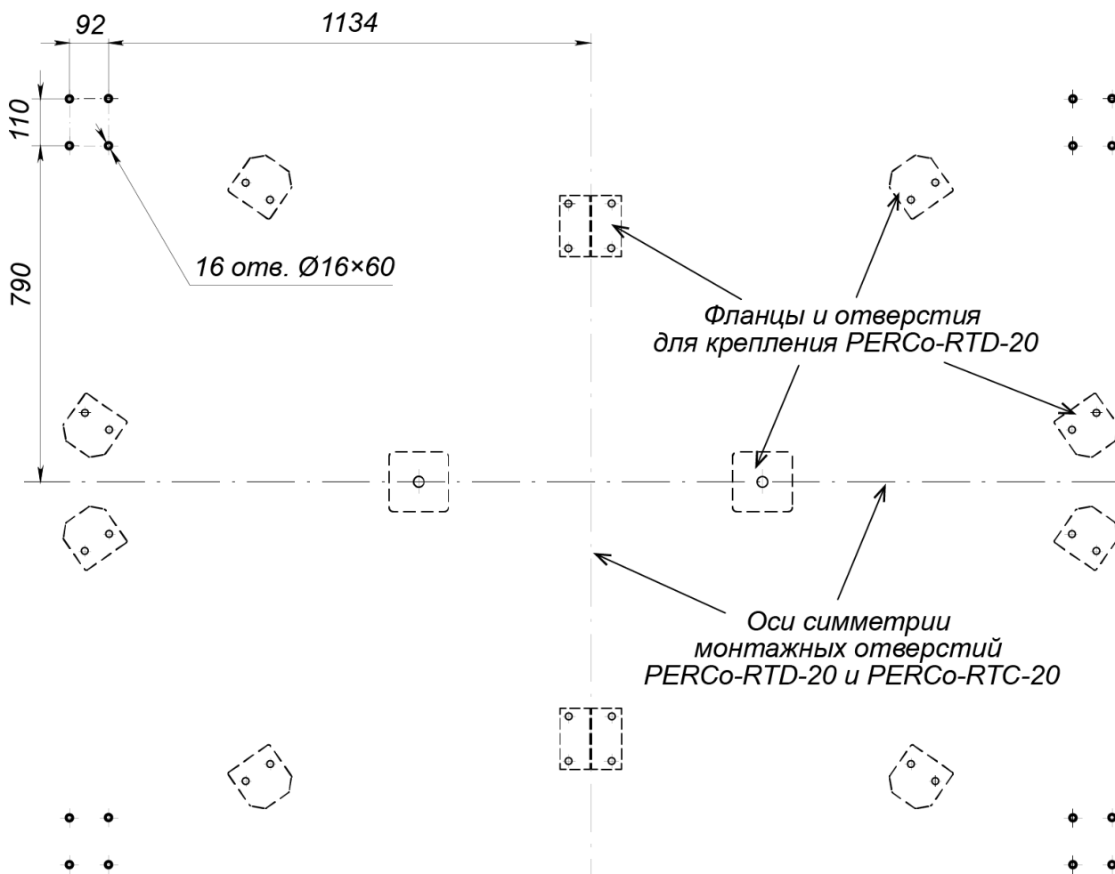
Рисунок 3. Схема разметки отверстий для установки крыши PERCo-RTC-20 1
