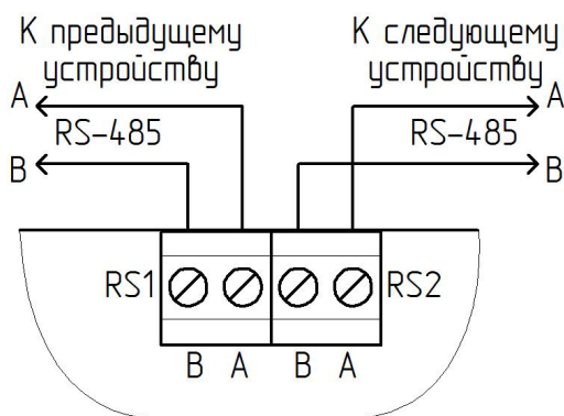
Рисунок 8 – Подключение RS-485
