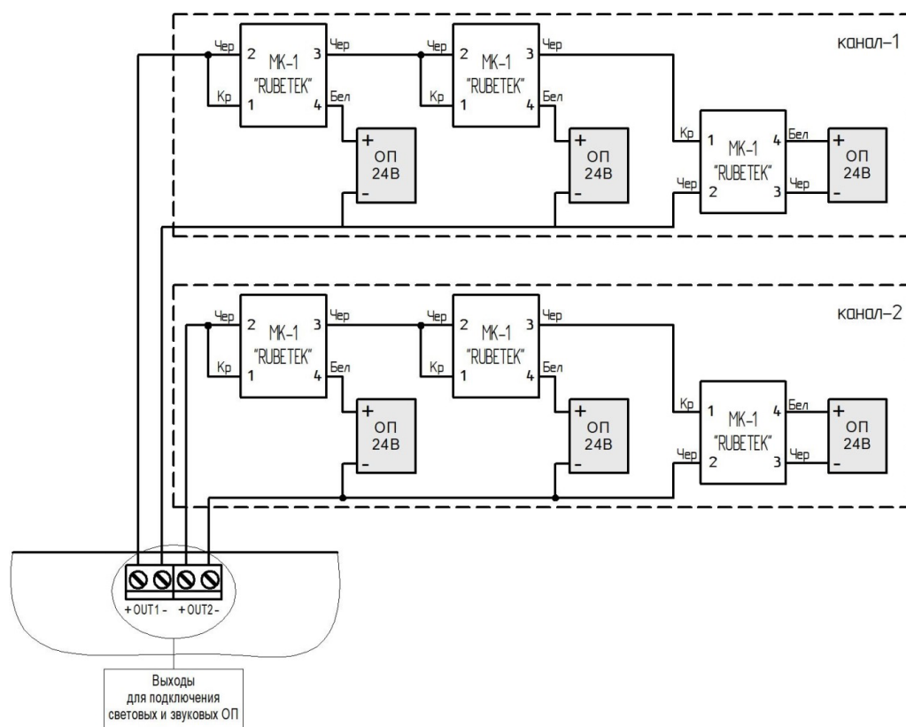
Рисунок 11 – Схема подключения СОУЭ
