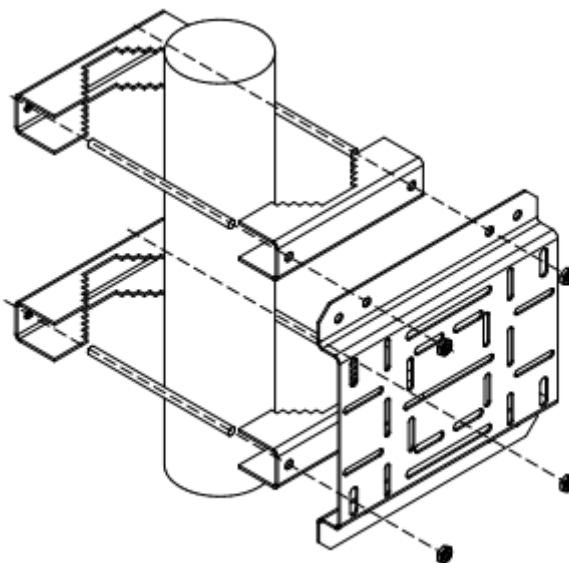
Рис.4. Схема сборки
