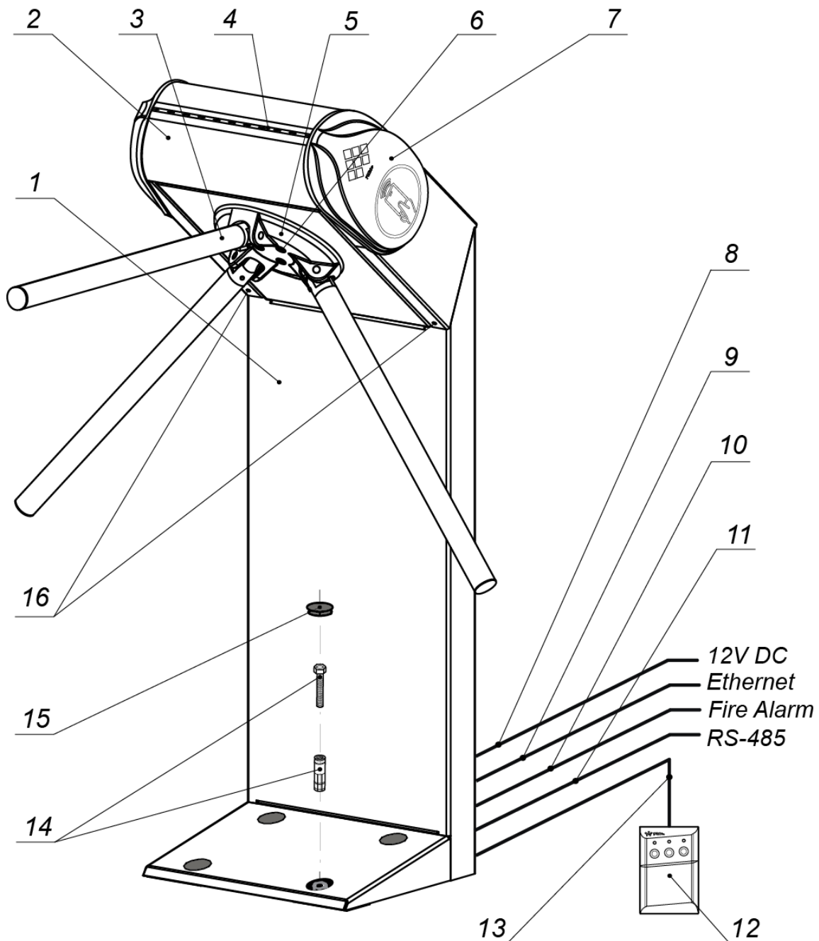
Рисунок 1. Устройство ЭП
