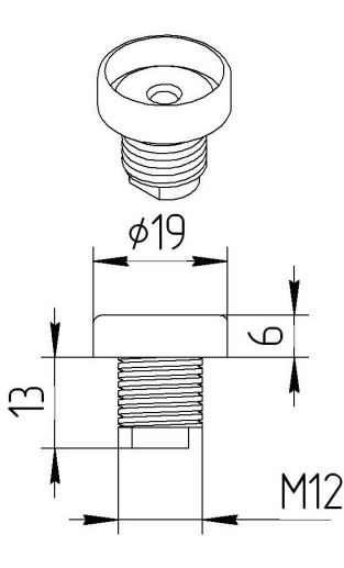
Рис.2 Контактор КТВС
