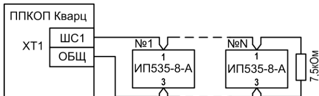
Рис.А6 Схема подключения ручных пожарных извещателей ИП535-8-А
