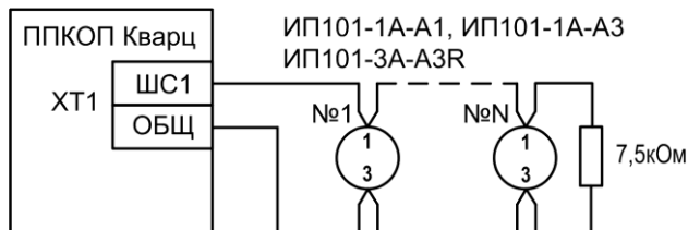
Рис.А5 Схема подключения тепловых пожарных извещателей ИП101-1А-А1(А3), ИП101-3А-А3R
