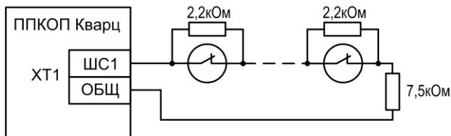
Рис.А7 Схема подключения тепловых пожарных извещателей типа ИП103, ИП105
