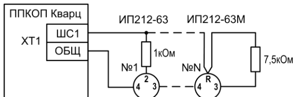
Рис.А4 Схема подключения дымовых пожарных извещателей ИП212-63 «ДАНКО» и ИП212-63М «ДАНКО вариант 2»
