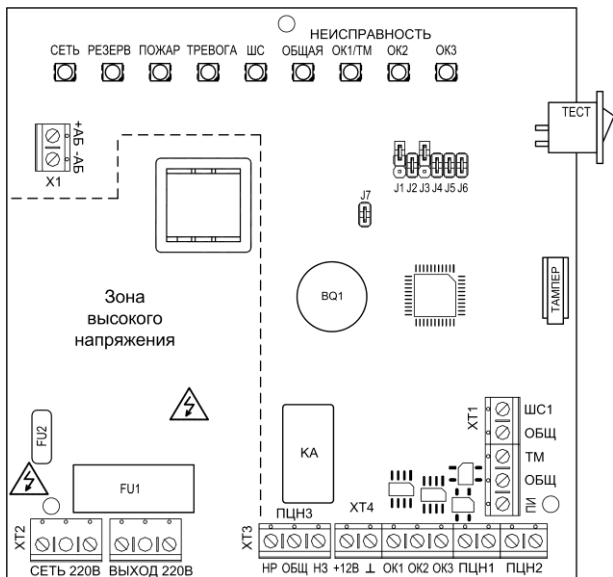
Рис.3 Плата прибора
