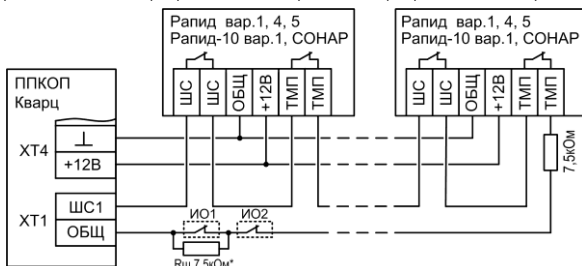
Рис.А9 Схема подключения охранных извещателей Рapid вар.1,4,5, Rapid-10 вар.1, СОНАР, ПОЛЮС-2 (ИО1, ИО2)
