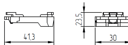
Масса – 0,006 кг Рисунок А.6 – Монтажное основание OptiSignal D22 A5-MB
