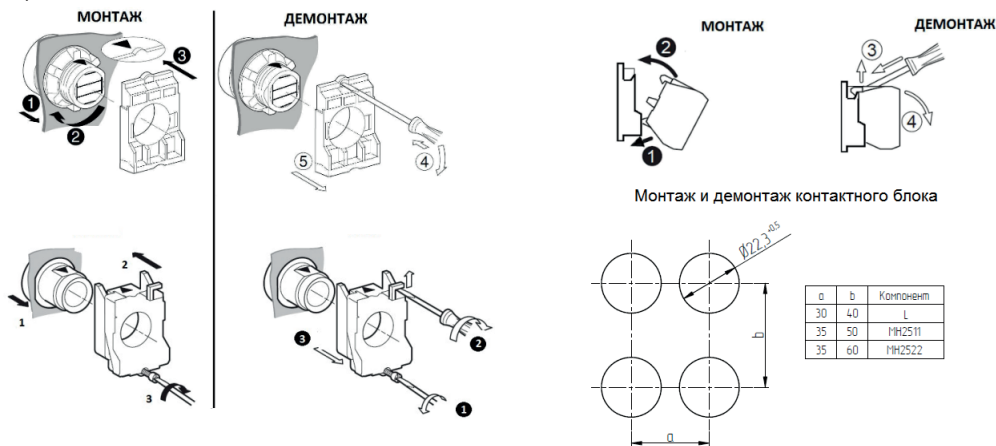
Рисунок 1 – Схема монтажа и демонтажа ламп
