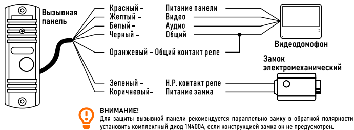
Схема подключения вызывной панели к домофону и электромеханическому замку
