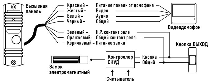
Схема подключения вызывной панели к домофону, контроллеру СКУД и электромагнитному замку
