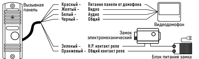
Схема подключения вызывной панели к домофону и электромеханическому замку
