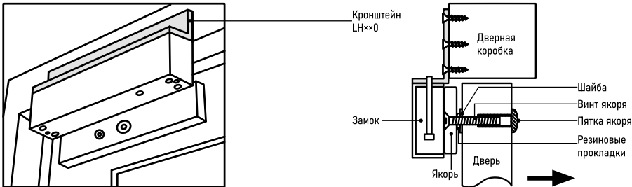
Рис. 1 Монтаж с помощью кронштейна L-типа (LHxx0)
