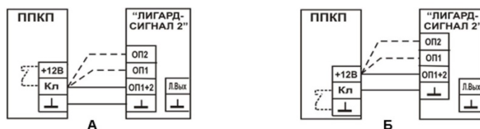
Рис.3 Монтажные схемы Лигард-Сигнал-2
