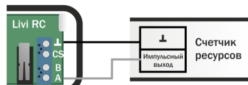
Рисунок 7.3 – Схема подключения датчика к одному счетчику электроэнергии или воды
