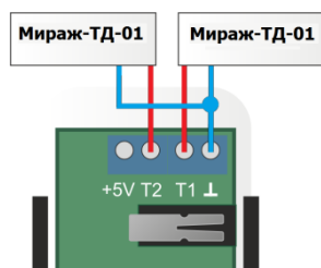
Рисунок 8.2 – Схема подключения внешних сенсоров Мираж-ТД-01
