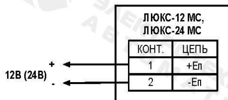
Рис.1. Схема подключения.
