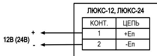
Рис.1. Схема подключения.
