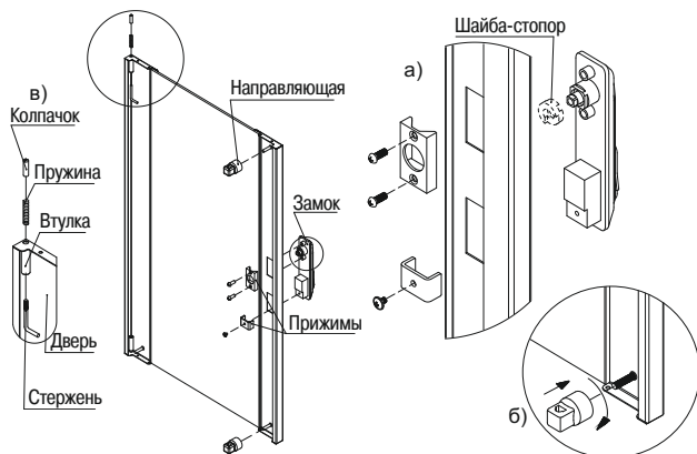
Рисунок 11 – Сборка дверей
