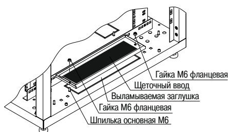
Рисунок 16 – Монтаж щеточного ввода
