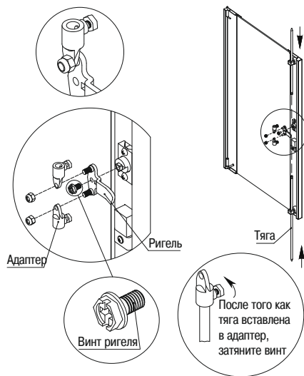
Рисунок 12 – Сборка дверей
