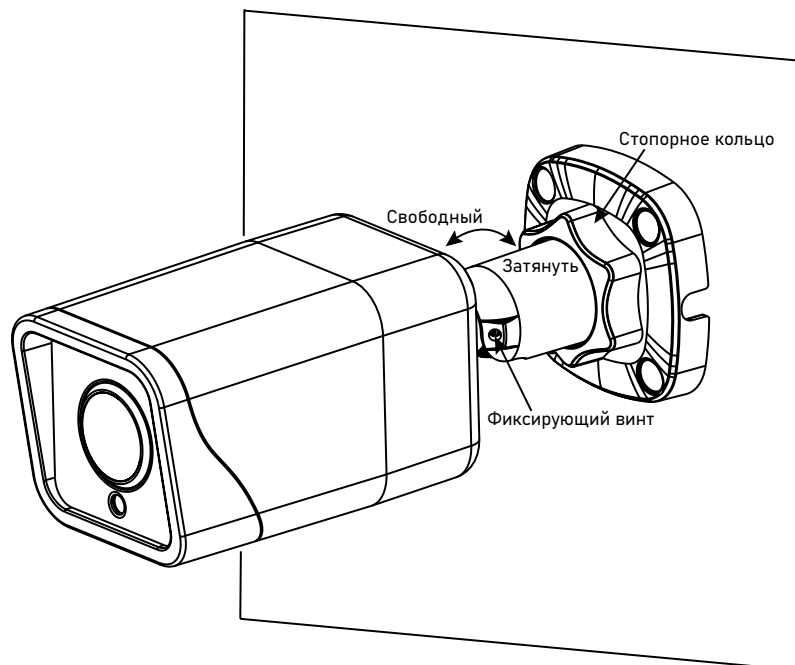
Рис. 12. Направление обзора камеры
