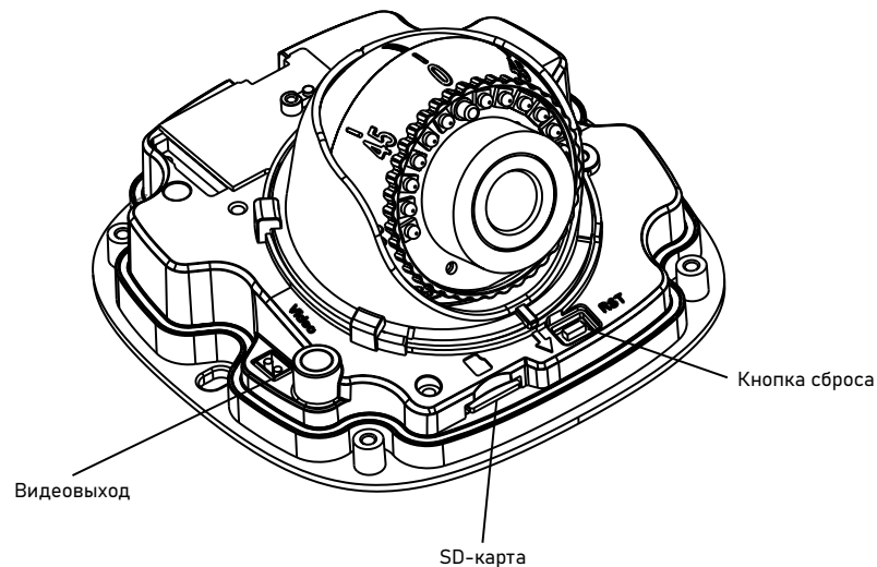
Рис. 26. Подключение кабелей
