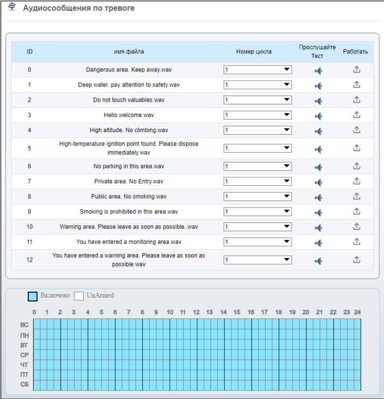
Рис. 87. Аудиосообщения по тревоге
