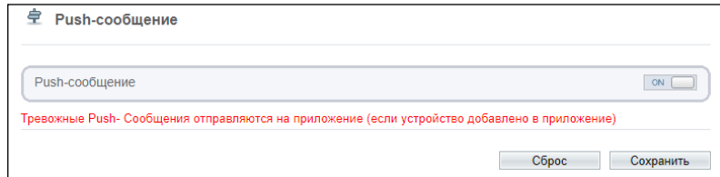
Рис. 86. PUSH-сообщение
