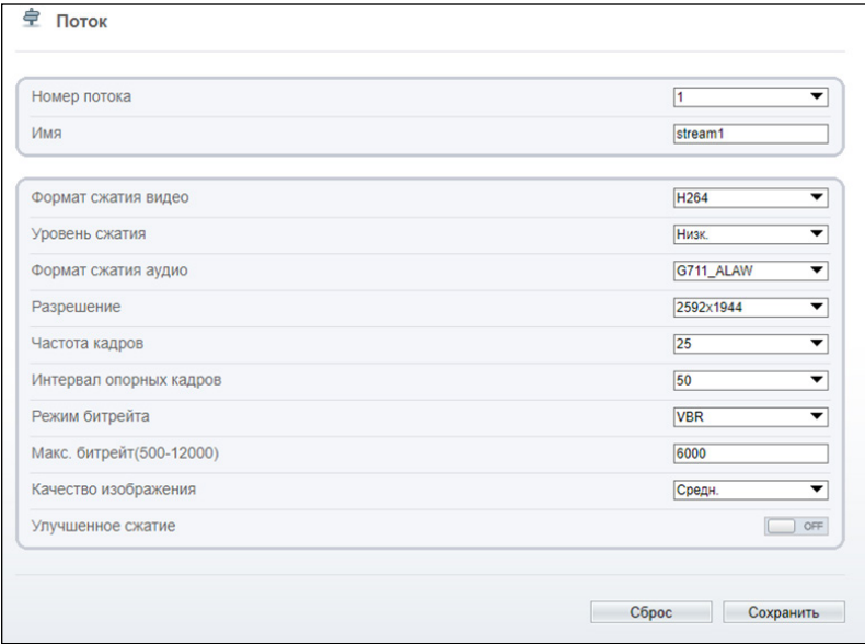
Рис. 57. Настройки видео/аудио потоков
