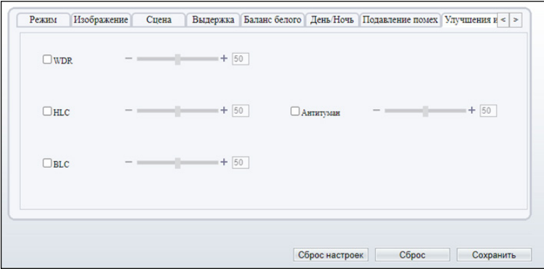
Рис. 54. Улучшения изображения
