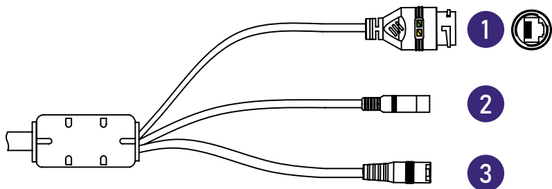
Рис. 19. Подключение кабелей
