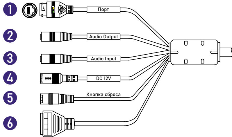
Рис. 1. Подключение кабелей
