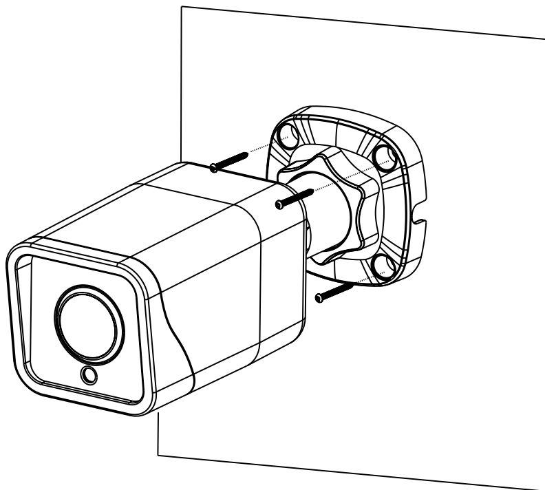
Рис. 11. Монтаж камеры
