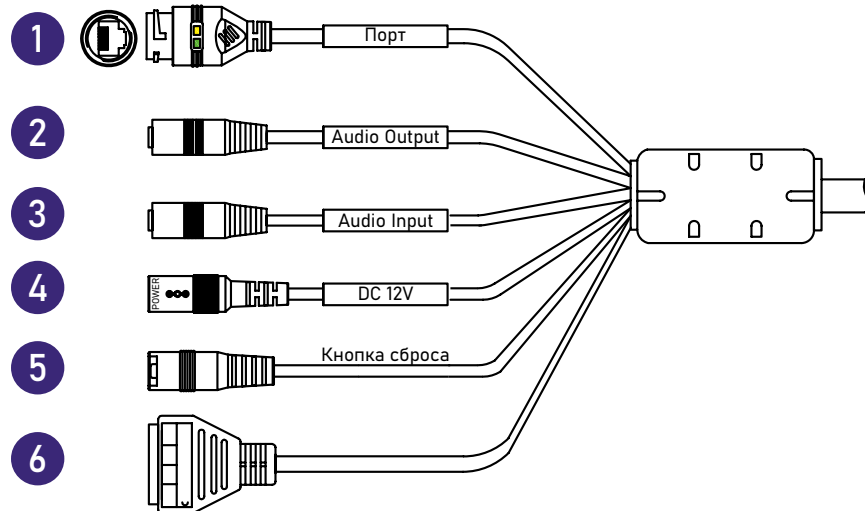
Рис. 13. Подключение кабелей
