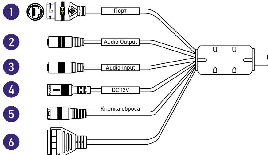
Рис. 25. Подключение кабелей
