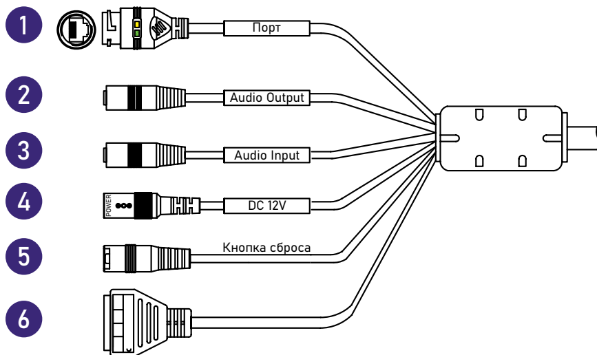
Рис. 7. Подключение кабелей
