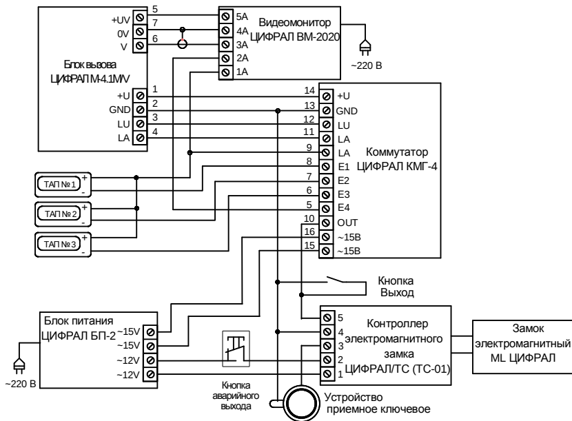
Рисунок В.3 Схема подключения домофонов ЦИФРАЛ М-4.1М/В
