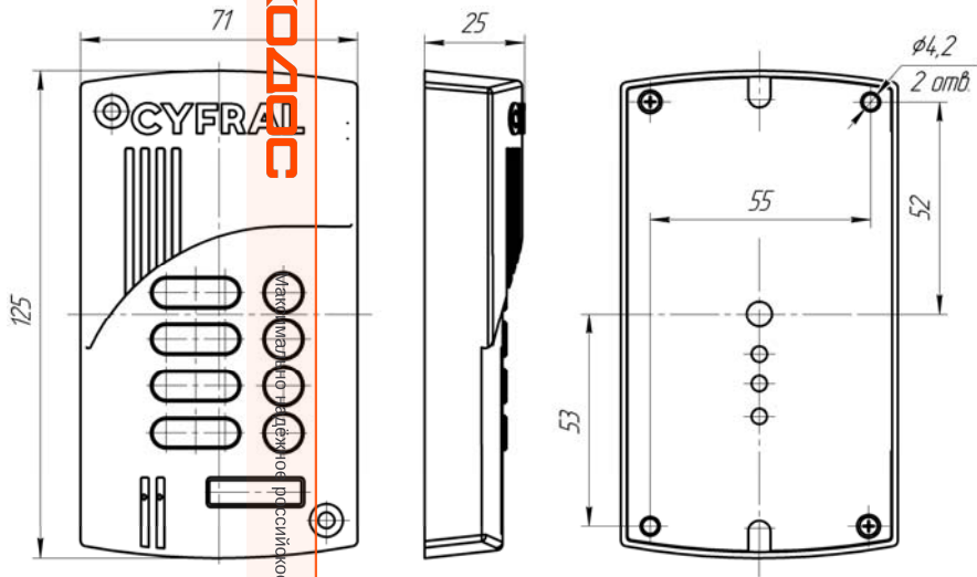
Рисунок А.2 Установочные и габаритные размеры блока вызова ЦИФРАЛ М-4.1М (ЦИФРАЛ М-4.1М/V, ЦИФРАЛ М-4.1М/VC)
