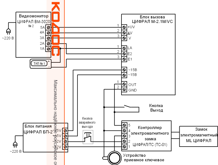
Рисунок Б.2 Схема подключения домофона ЦИФРАЛ М-2.1М/ВС
