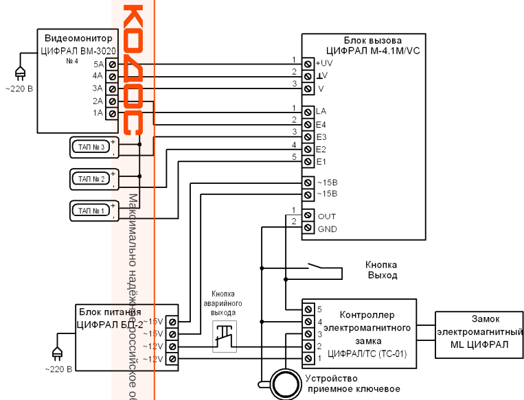
Рисунок Б.4 Схема подключения домофона ЦИФРАЛ М-4.1М/VC
