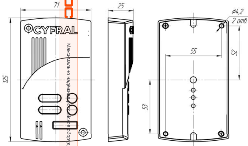
Рисунок А.1 Установочные и габаритные размеры блока вызова ЦИФРАЛ М-2.1М (ЦИФРАЛ М-2.1М/V, ЦИФРАЛ М-2.1М/VC)
